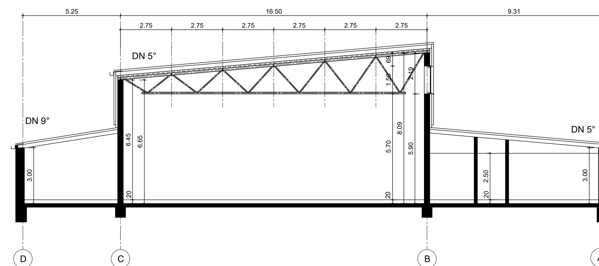
Systemschnitt
